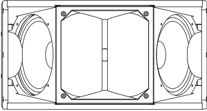
Fig. 1: Q1 loudspeaker
